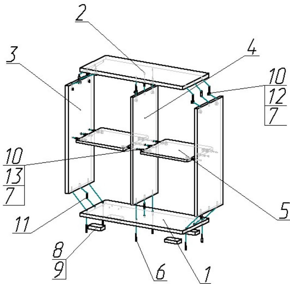
Рис. 1 Сборка стеллажа
