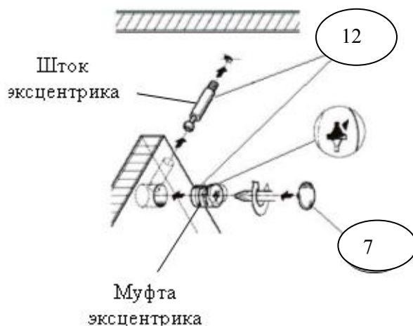
Рис. 1 Сборка стеллажа
